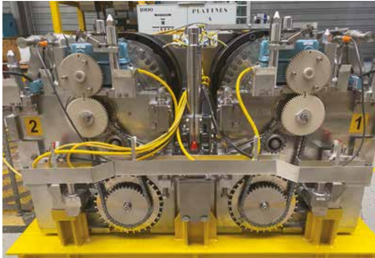
Unité de levage sécurisée 50 kN en cellule chaude pour l'usine de La Hague
