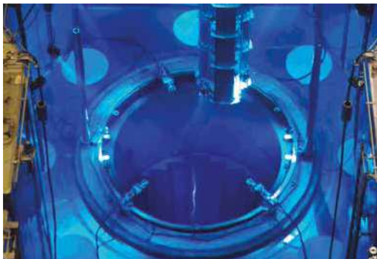
Outillage vidéo bord de cuve
