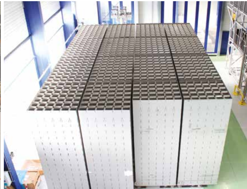
Rack de stockage du combustible usé (RSCU)
